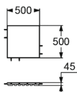
КОВРИК РЕЗИНОВЫЙ ПРЯМОЙ (толщина 45 мм)
