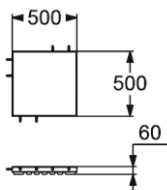
КОВРИК РЕЗИНОВЫЙ ПРЯМОЙ (толщина 60 мм)
