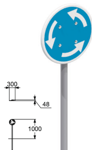
6848 ДОРОЖНЫЙ ЗНАК "КРУГОВОЕ ДВИЖЕНИЕ"
