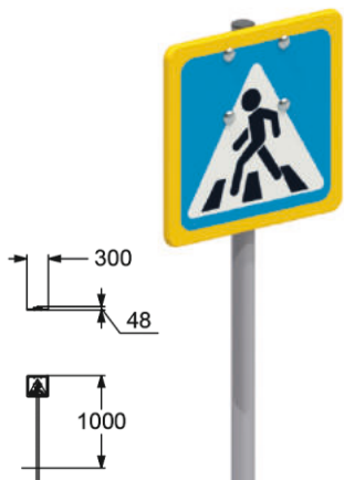
6841 ДОРОЖНЫЙ ЗНАК "ПЕШЕХОДНЫЙ ПЕРЕХОД"
