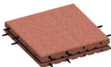
КОВРИК РЕЗИНОВЫЙ ДВУХСЛОЙНЫЙ (толщина 105 мм)
