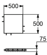
КОВРИК РЕЗИНОВЫЙ ДВУХСЛОЙНЫЙ (толщина 75 мм)
