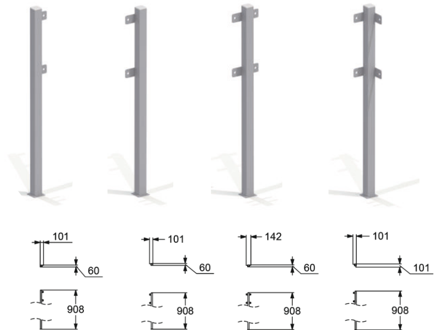
2770 СТОЙКА ДЛЯ ОГРАЖДЕНИЯ
