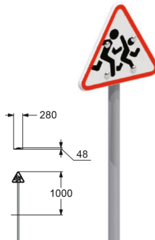
6843 ДОРОЖНЫЙ ЗНАК "ДЕТИ"
