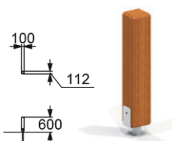
2780 СТОЙКА ДЕКОРАТИВНОГО ОГРАЖДЕНИЯ
