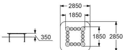
2455 ДОРОЖКА "МАЛЫЙ КВАДРАТ"
