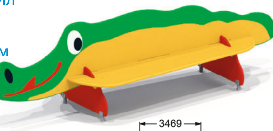
2409 СКАМЕЙКА ДЕТСКАЯ "КРОКОДИЛ"
