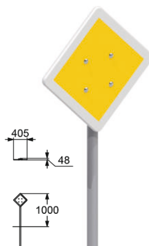
6847 ДОРОЖНЫЙ ЗНАК "ГЛАВНАЯ ДОРОГА"
