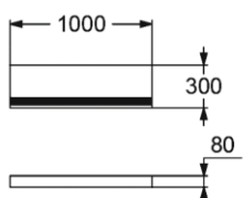
БОРДЮР РЕЗИНОВЫЙ (толщина 80 мм)
